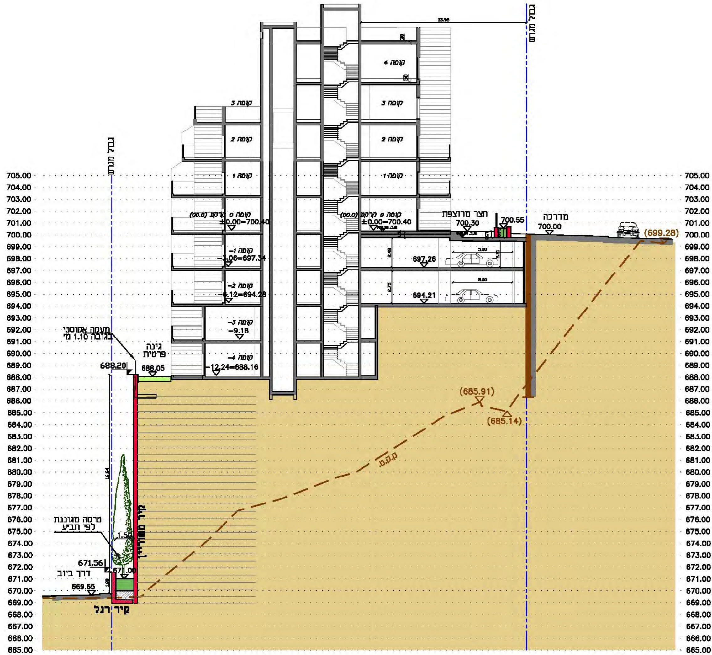
חתך ו-1
