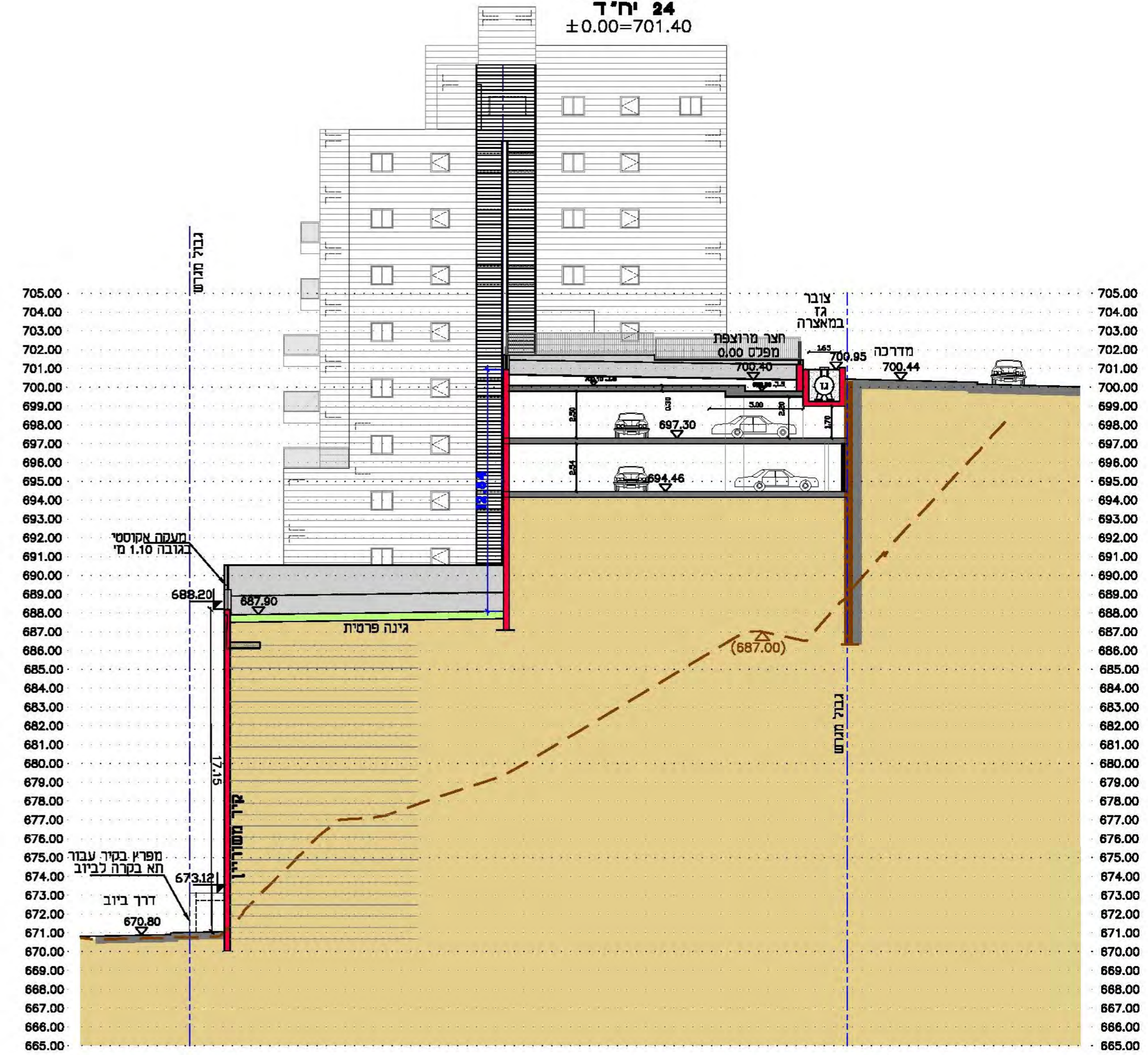
חתך ו-א-א
